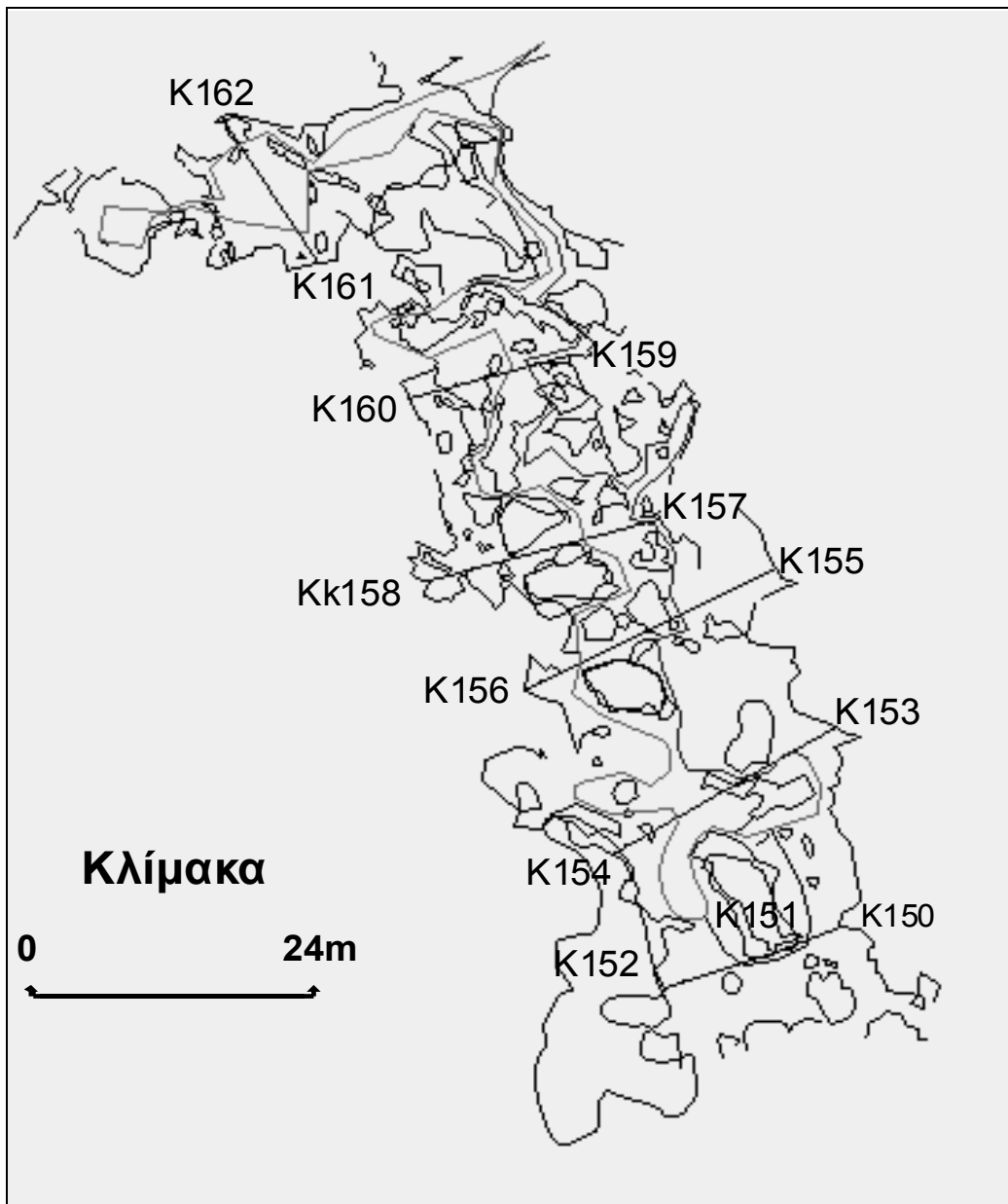
Σχήμα 7. Οριζοντιογραφία σπηλαίου με τις εξεταζόμενες διατομές (Σύμφωνα με το τοπογραφικό σχέδιο του Τοπογράφου Δ. Πετριδη, γραφείο τοπογραφικών εφαρμογών «ΓΕΩΓΡΑΦΕΙΝ», Αλεξανδρούπολη).
