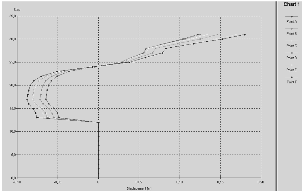
Εικόνα 5. Γραφική παράσταση των μετακινήσεων των κόμβων που αντιστοιχούν στις θέσεις των μαγνητικών πλάκων του οριζόντιου idel\ HI - 4 σε συνάρτηση με τα υπολογιστικά βήματα της διαδικασίας προσομοίωσης.
